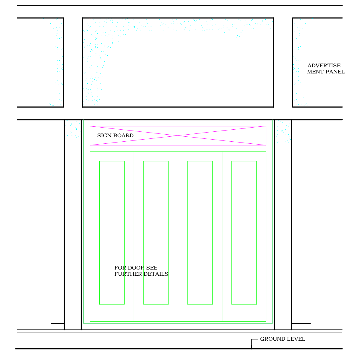
ELEVATION
