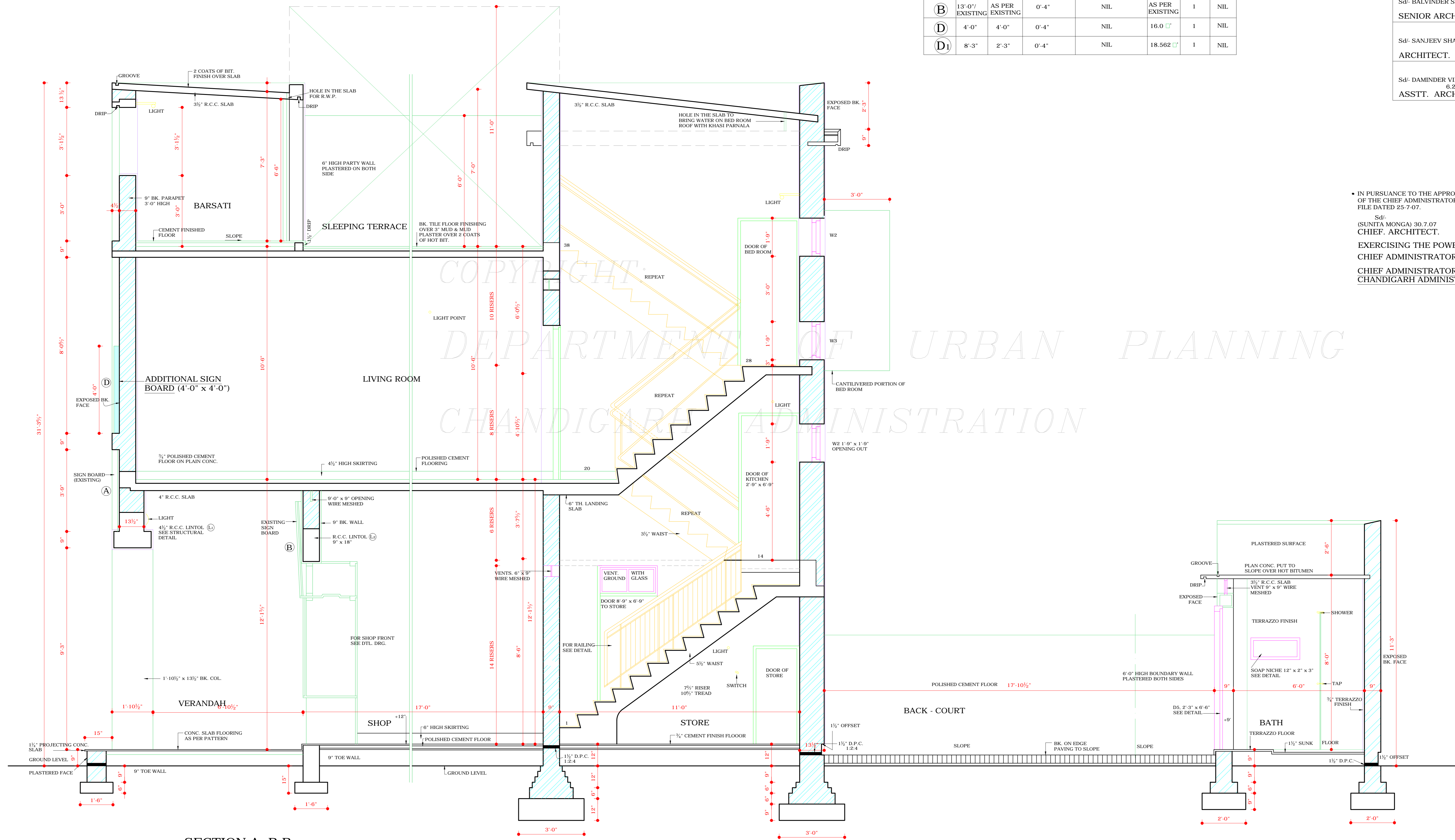
SECTION A: B-B
